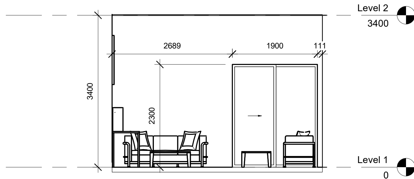
1 Elevation 1 1 : 50
