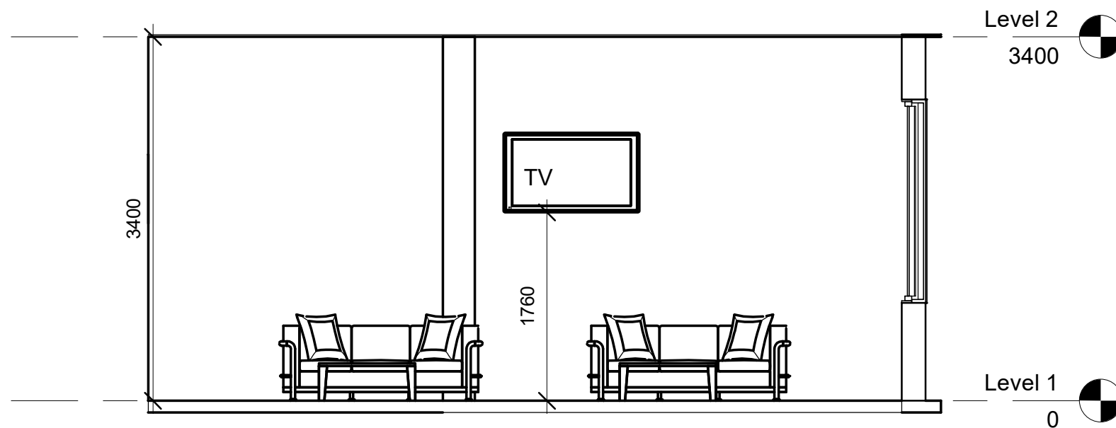
2 Elevation 2 1 : 50
