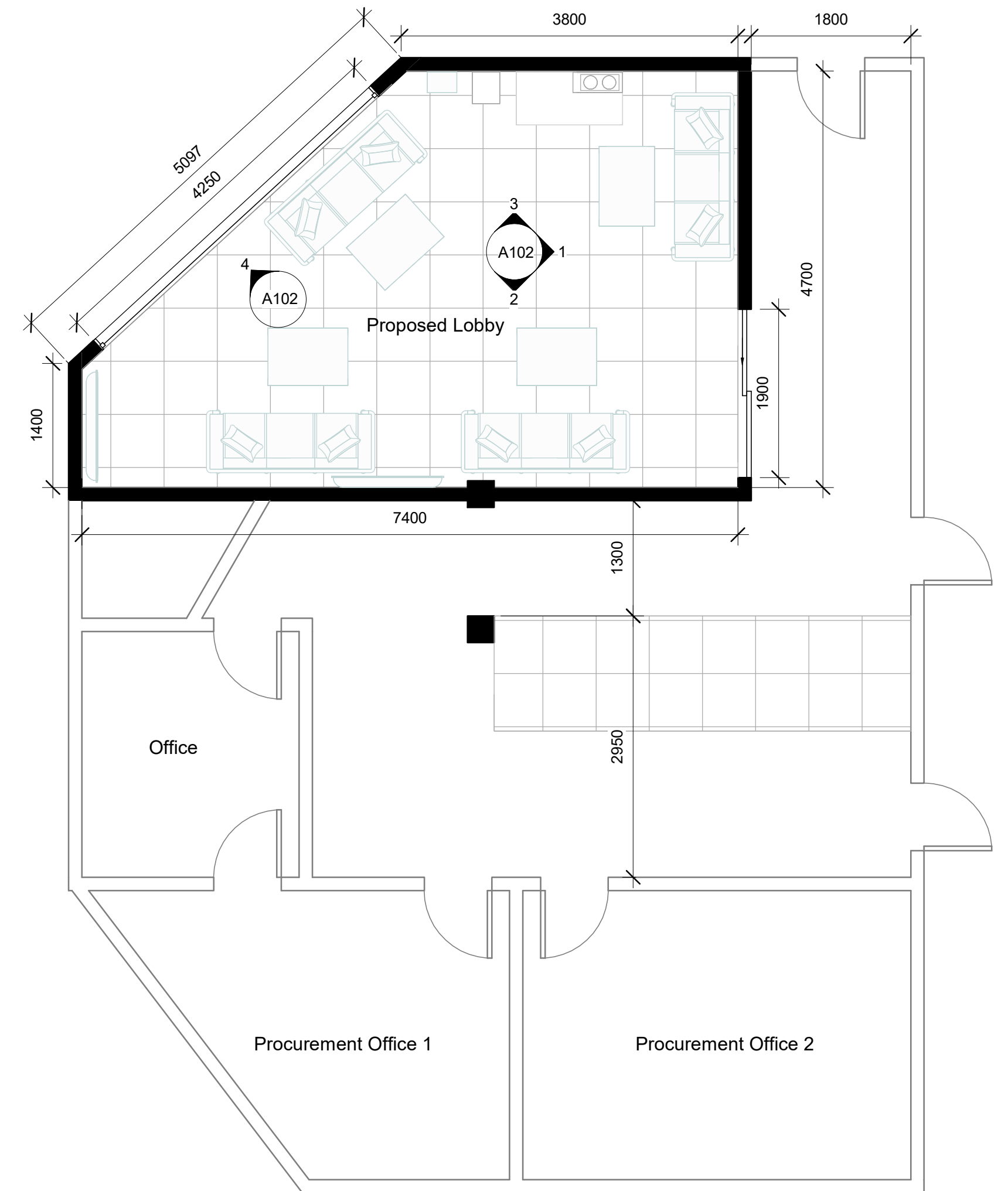
1 Floor Level 1 : 50
