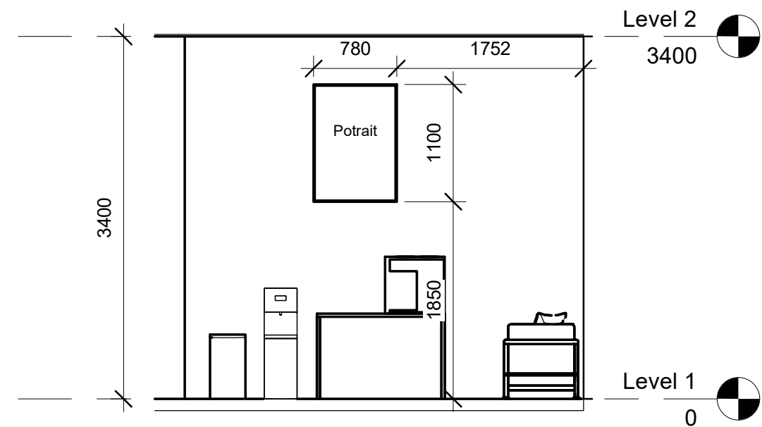
3 Elevation 3 1 : 50
